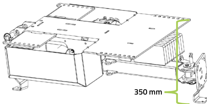
Abbildung 7 – Tiefe (Ohne Lader-Aufnahme): PUMA 2803-Multiträger
