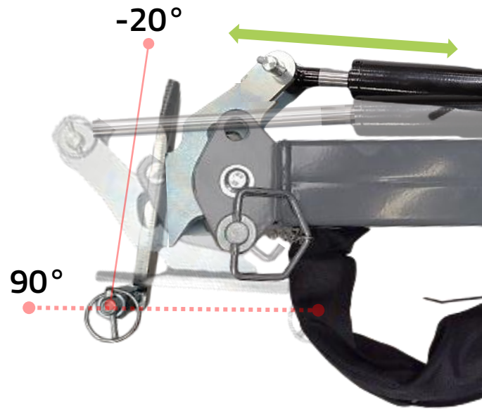
Hydraulische Schnitzwinkelverstellung am PUMA 2803 Multiträger
