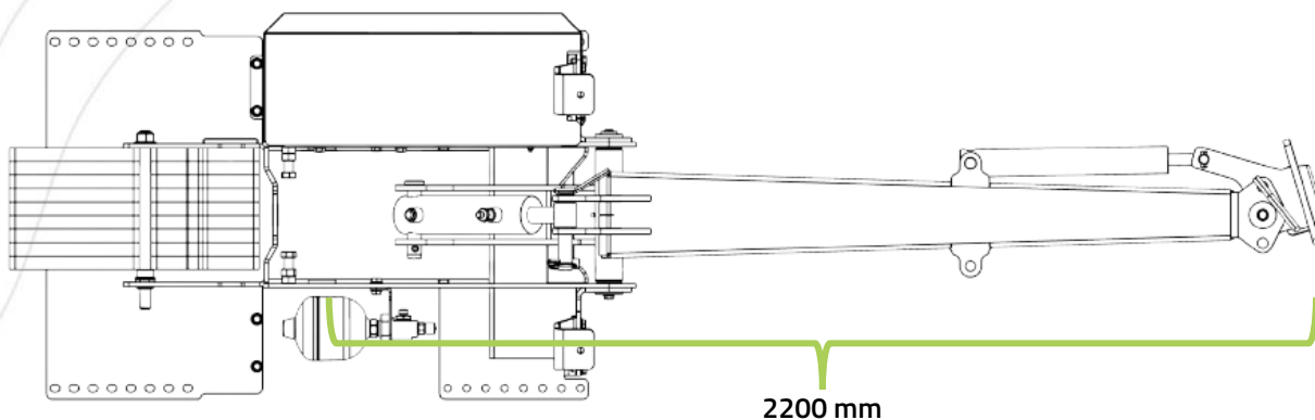
Abbildung 9 – Reichweite in Arbeitsposition (ab Maschinenmitte ohne Anbaugerät): PUMA 2803-Multiträger
