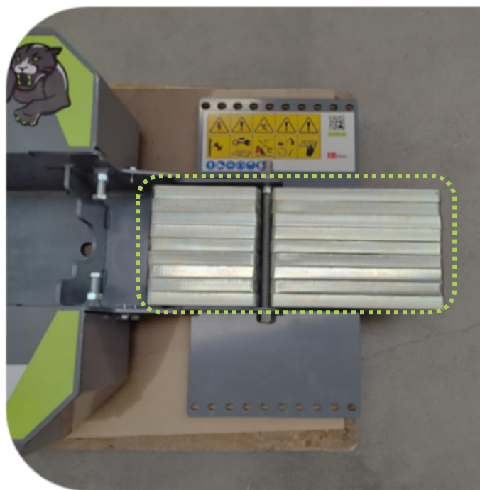
Gegengewichte (85 kg), montiert auf PUMA 2803 Multiträger
