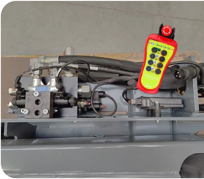
Ölmengenteiler m. E-Bedienung: PUMA 2803 Plus Multiträger
