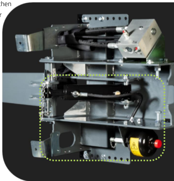
Akkumulator mit Anfahrzylinder verbunden
