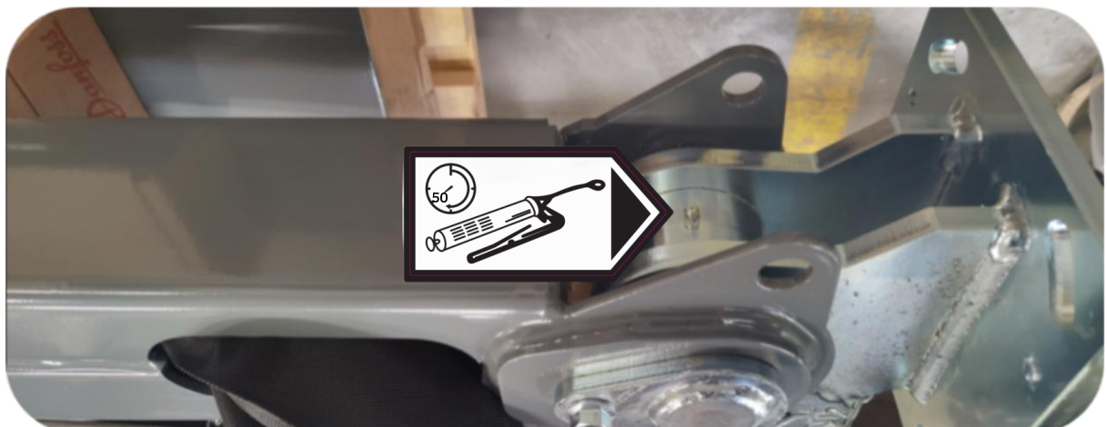
Position des Schmiernippels am Ende des PUMA 2803-Multiträger-Schwenkarms
