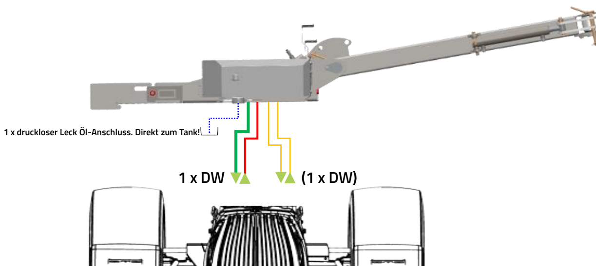
Hydraulikschlauchverbindungen zwischen PUMA 2803-Multiträger und Fahrzeug
