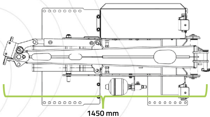
Abbildung 8 – Transportbreite (ohne Anbaugerät): PUMA 2803-Multiträger
